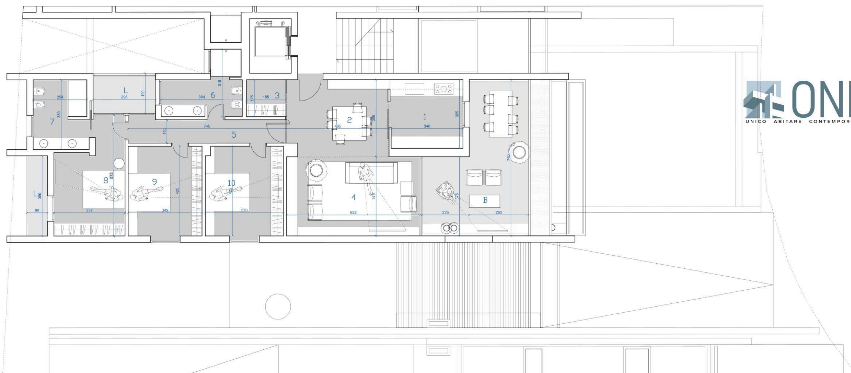
PIANTA LIVELLO TERZO | ALLOGGIO 7 SCALA 1:100
