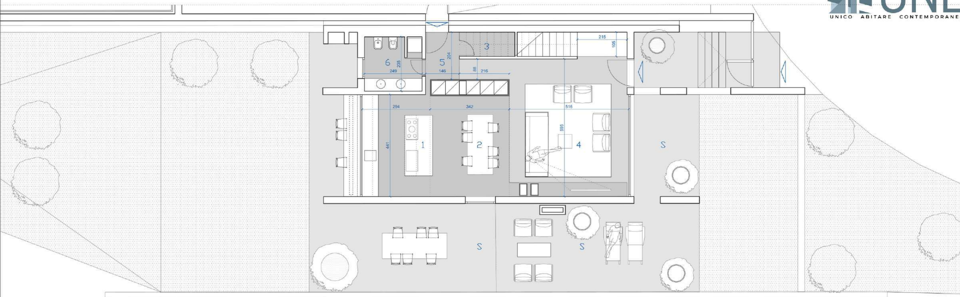
PIANTA LIVELLO TERRA | ALLOGGIO 1 SCALA 1:100
